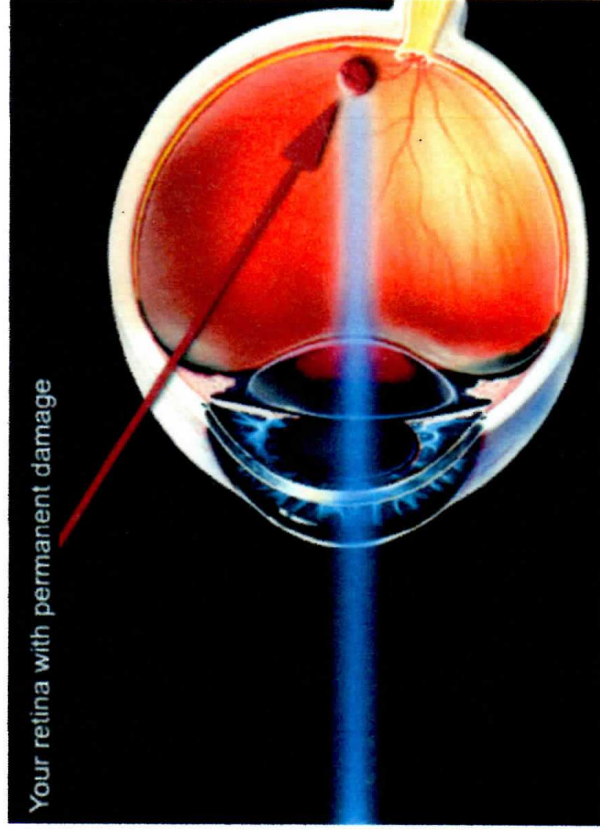
El ojo humano con un alargamiento esquemático de la retina
